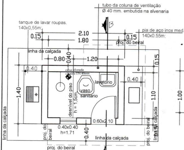
PLANTA BAIXA
