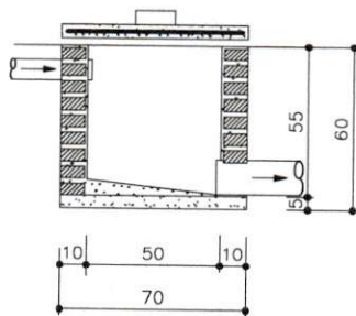
CORTE AA
